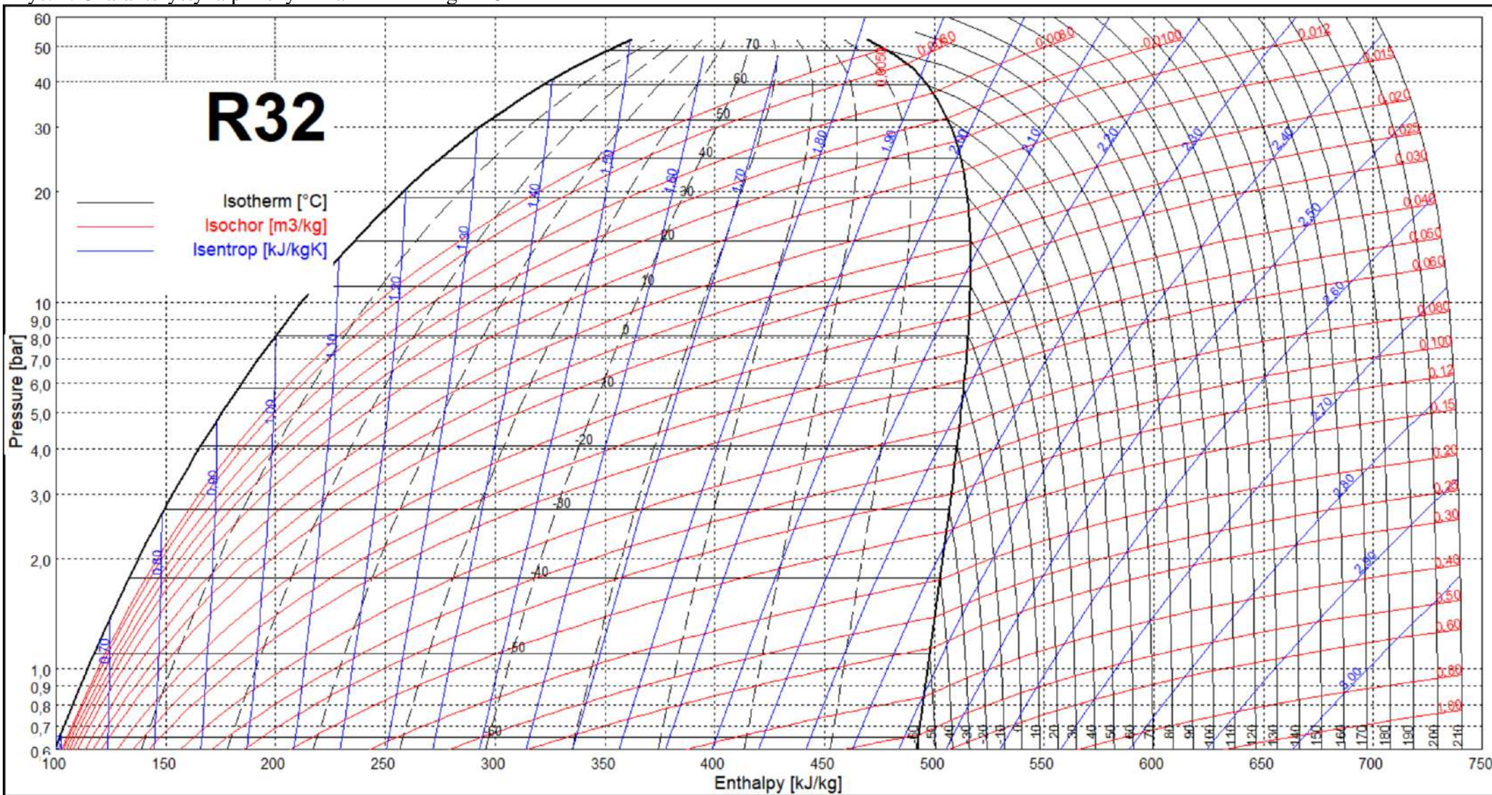
Rys. 2. Charakterystyka p-h czynnika chłodniczego R 32
