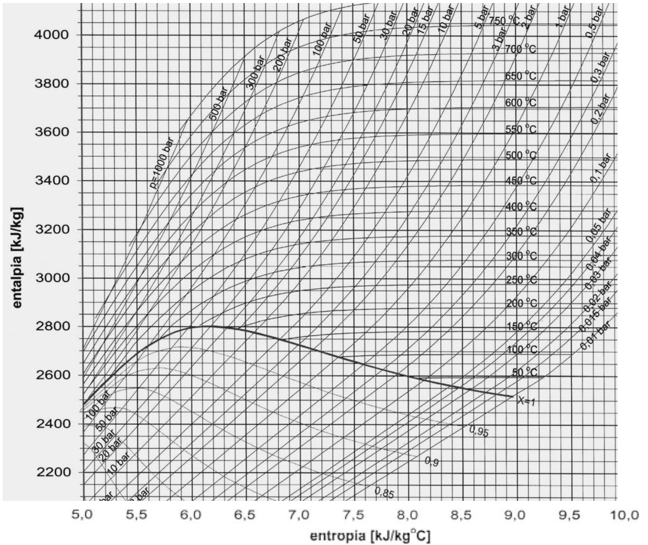
Rys. 3. Wykres i-s dla pory wodnej – fragment pola roboczego
